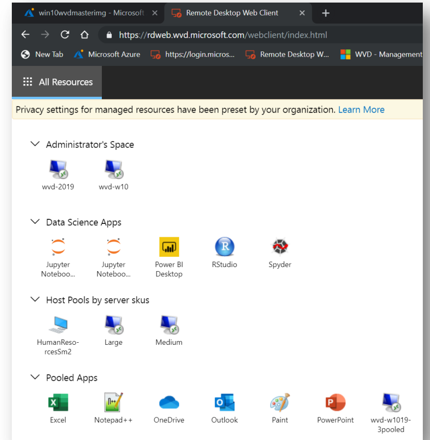
HTML 5 Browser
